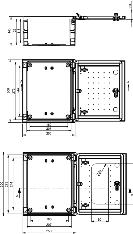
EPC/EPC-W 30-25-14
